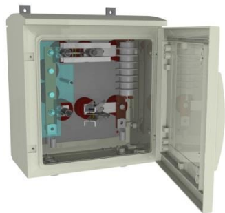
IC MDI 3.6kV 1250A 2IN + 1OUT + SVL
